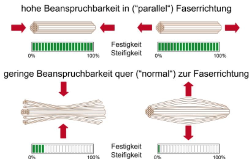
Abb. 2: Beanspruchbarkeit von Holz in Abhängigkeit zur Faserrichtung [2]
