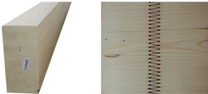
Abb. 3: Brettchichtholz; Keilzinkung einer BSH-Lamelle
