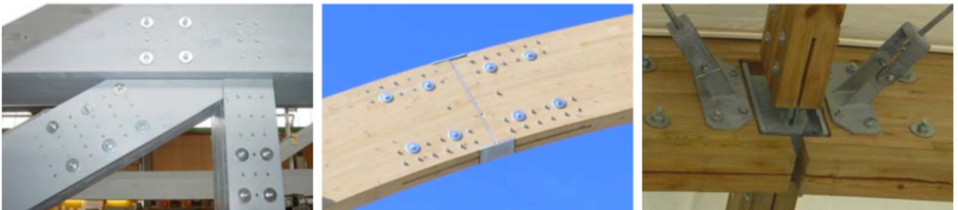
Abb. 7: Knoten und Montagestoß mit eingeschlitzten Stahlblechen, Stahlformteilen sowie Stabdübel und Passbolzen
